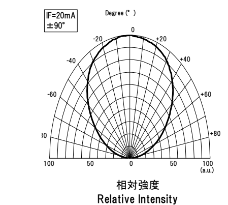
■ 指向性 Directivity
