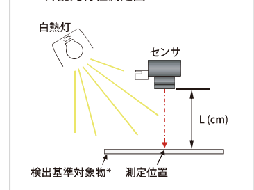
*1 外乱光特性測定図
