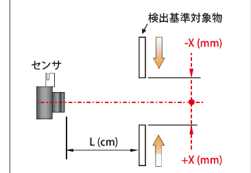
*2 検出範囲特性測定図
