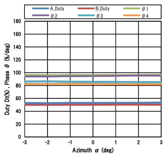
■ Duty・位相差/アジマス( \alpha )特性 Duty・Phase/Azimuth( \alpha ) Dependency
