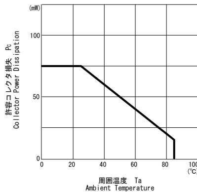
■コレクタ損失/周囲温度 P_c/T_a
