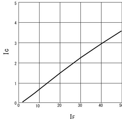
■ 光電流/順電流特性 Ic (mA) / If (mA)
