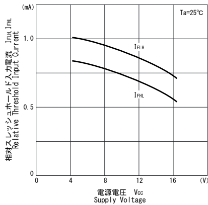
■相対スレッショールド入力電流/ 電源電圧特性 IF FLH , IF FHL /Vcc
