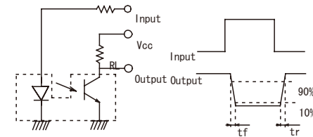
*1応答時間特性図
