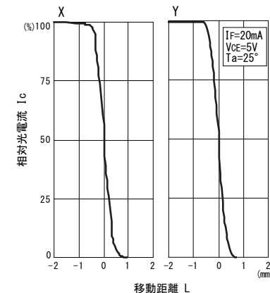
■ 位置検出特性 *2
