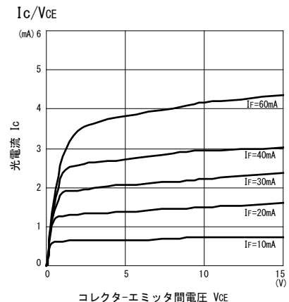
■ 光電流/コレクタ-エミッタ間電圧特性 I_c/V_{CE}
