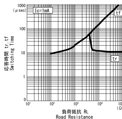
■ 応答時間/負荷抵抗特性 *1 tr, tf/RL
