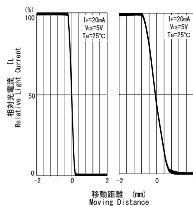
■位置検出特性 *2
