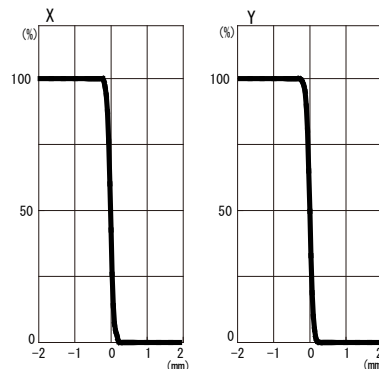
■ 位置検出特性 相対 I_c /移動距離 *2
