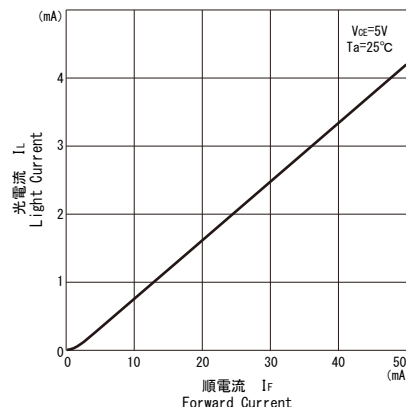
■光電流/順電流特性 I_L/I_F
