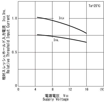
■ 相対スレッショールド入力電流 周囲温度特性 I_{FLH}, I_{FHL}/V_{CC}
