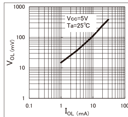
■ローレベル出力電圧/ローレベル出力電流特性 V OL (mV)/I OL (mA)
