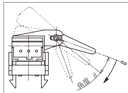
*1位置検出特性図
