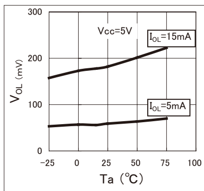
■ローレベル出力電圧/周囲温度特性 V OL (mV)/Ta(°C)
