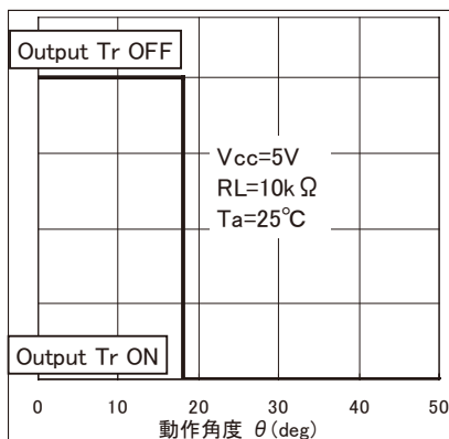
■位置検出代表特性 *1
