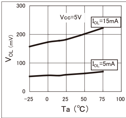
■ローレベル出力電圧/周囲温度特性 V_{OL}(mV)/T_a(^{\circ}C)
