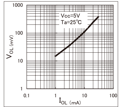
■ローレベル出力電圧/ローレベル出力電流特性 V_{OL}(mV)/I_{OL}(mA)
