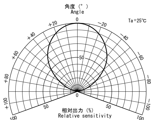
■指向特性
