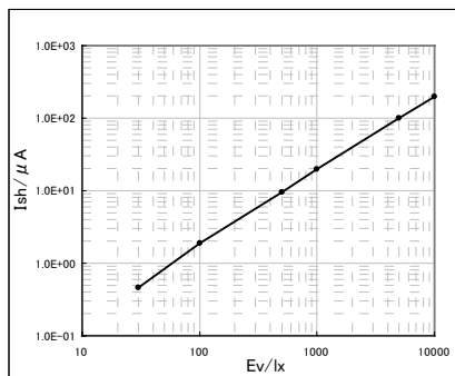
■ 短絡電流/照度特性 I_{sc}/E_v
