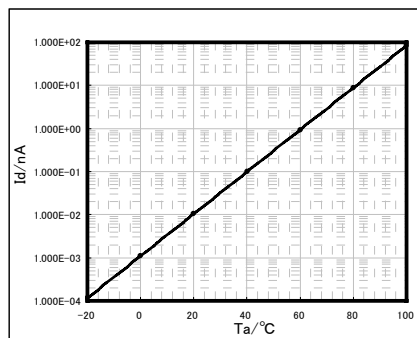
■ 暗電流/周囲温度特性 I_d/T_a
