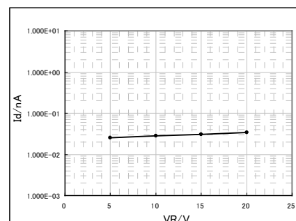
■ 暗電流/逆電圧特性 I_d/V_r
