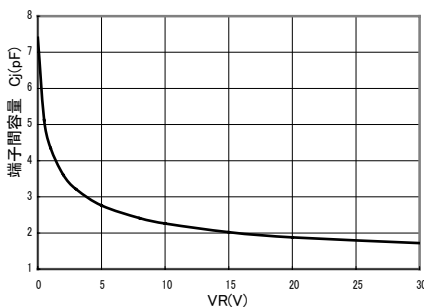
■ 端子間容量/逆電圧特性 C_t/V_r
