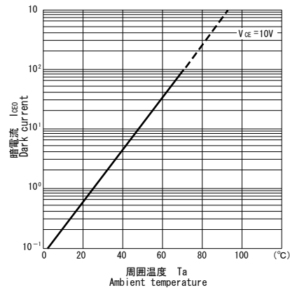
■暗電流/周囲温度特性 I_{CE0}/T_a (nA) 3
