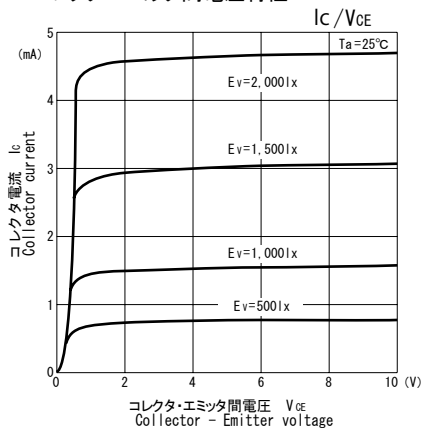
■コレクタ電流/ コレクタ・エミッタ間電圧特性
