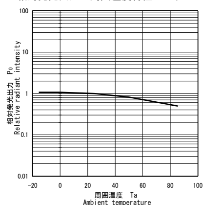
■相対発光出力／周囲温度特性 P_0/T_a
