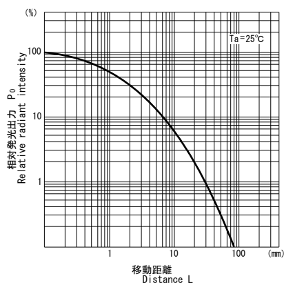
■相対発光出力／距離特性 P_o/L^{\ast 1}
