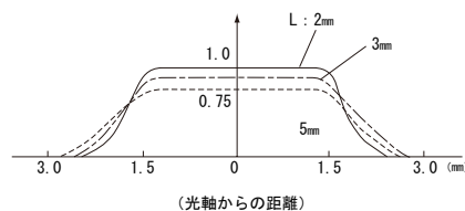
■相対光強度分布 ※2 RADIATION PATTERN
