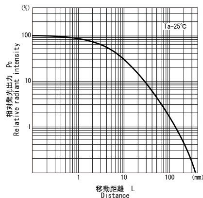
■相対発光出力／距離特性 P_0/L
