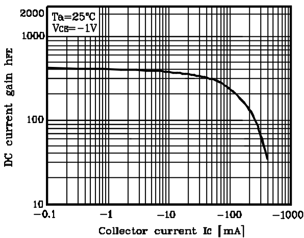
Fig. 3 h_{FE} - I_C
