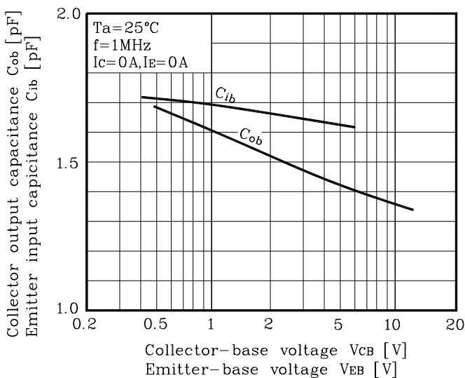
Fig. 5 C_{ob}-V_{CB}, C_{ib}-V_{EB}
