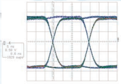
50Mbps発光波形 50Mbps transmitter waveform
